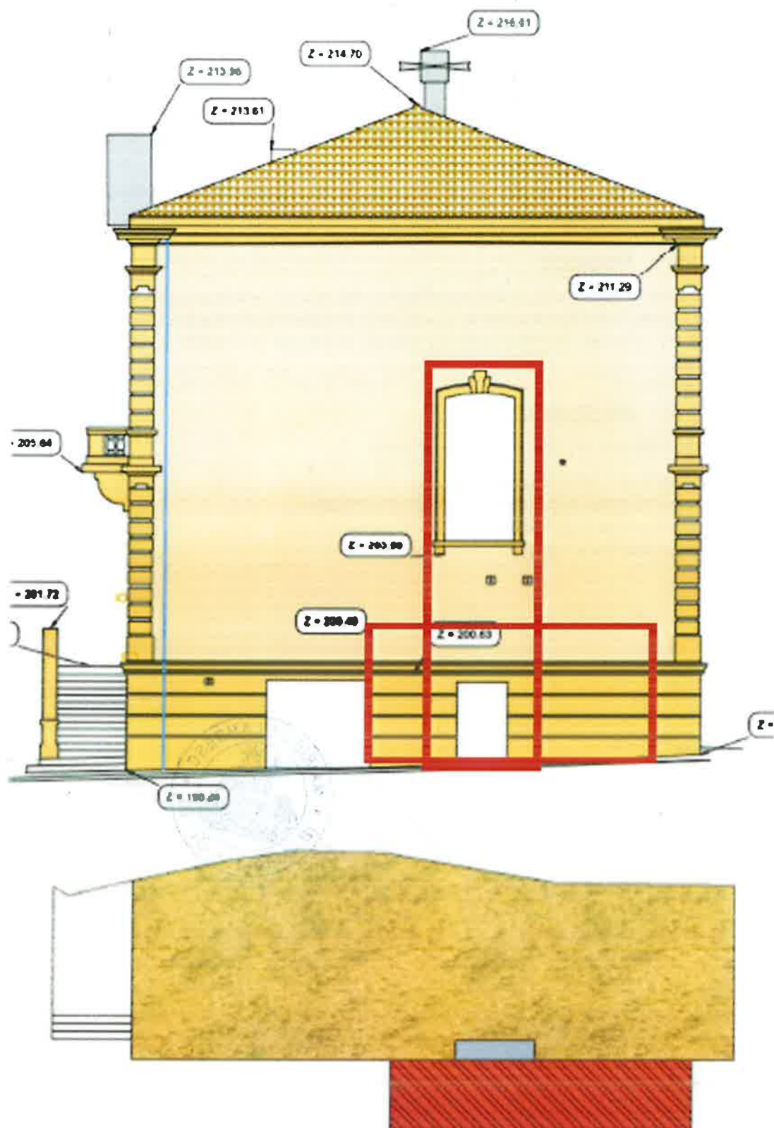
Emprise chantier rue du parage vue de dessus 1.5 m x 7m environ
